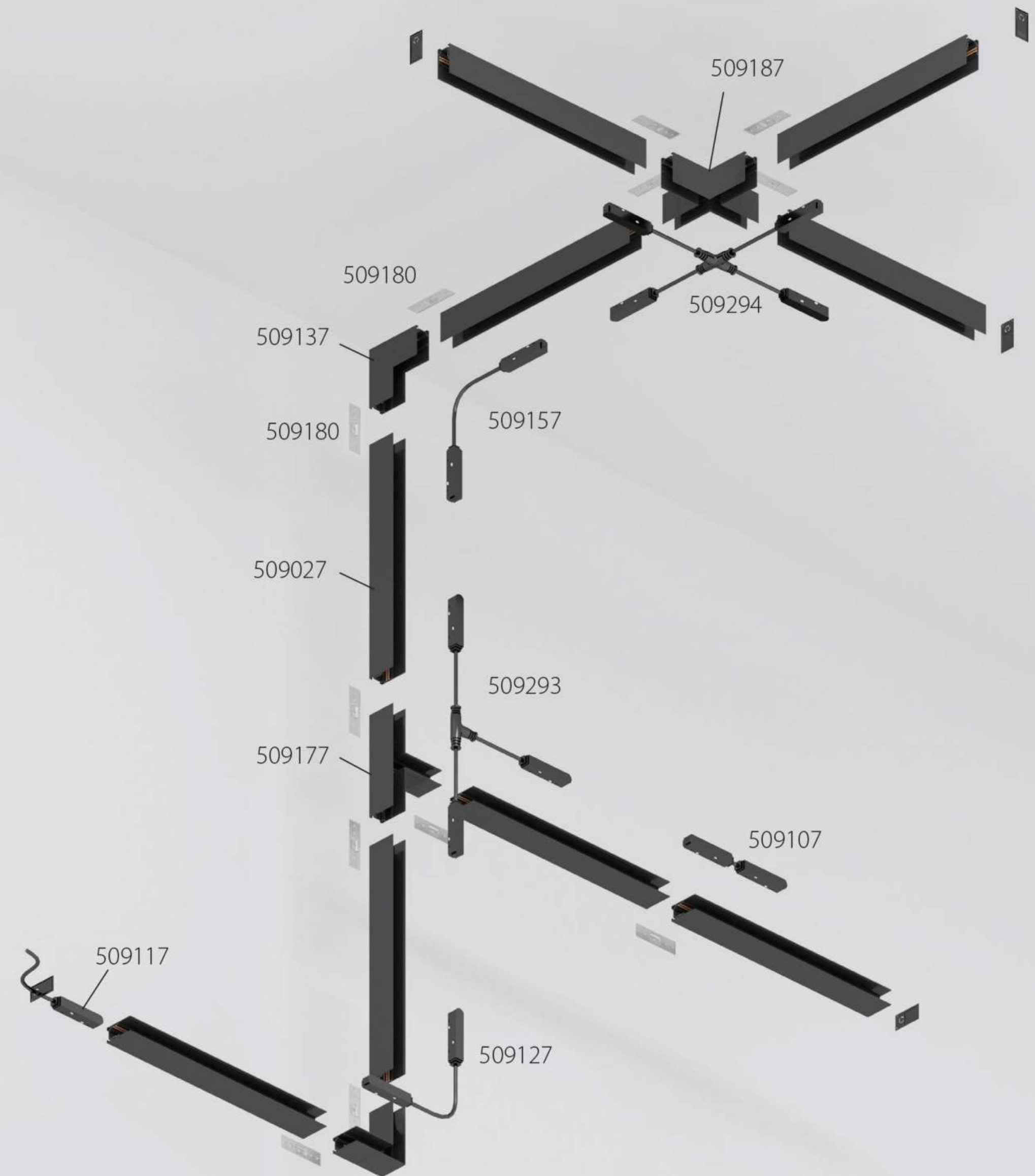
СХЕМА СБОРКИ ДЛЯ НАКЛАДНОГО ШИНОПРОВОДА
